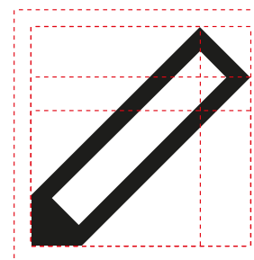
20_Mehrere_Zertifikate_verwalten_ Managed_PKI_SWS
